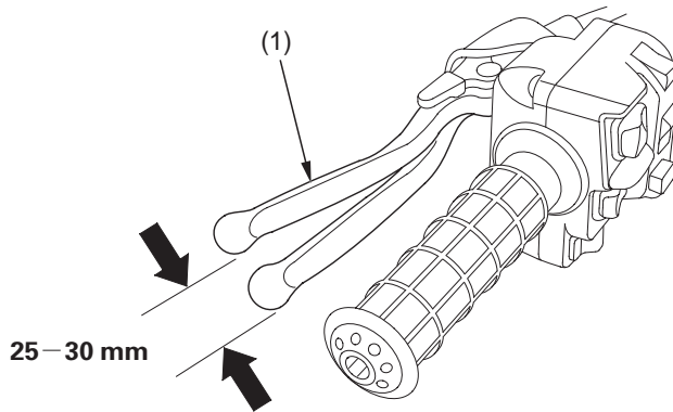
(1) takajarruvipu/pysäköintijarruvipu
